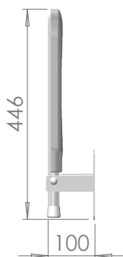
SZCZEGÓŁ A
